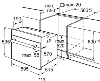
Рис.2 Размеры монтажа
