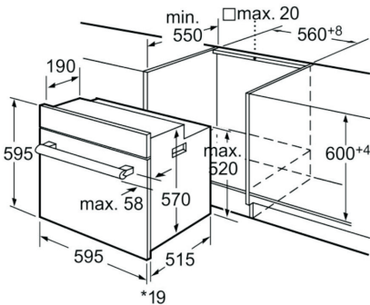
Мал.2 Розміри монтажу
