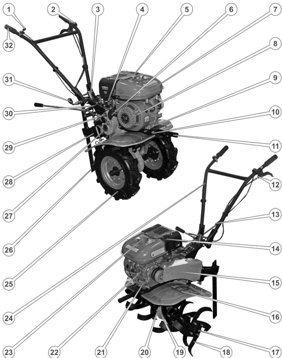
Рисунок 1.1. Елементи мотоблока
