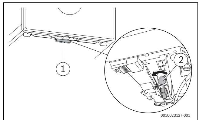
Мал. 4 Фіксування комунікаційного модулю Key
