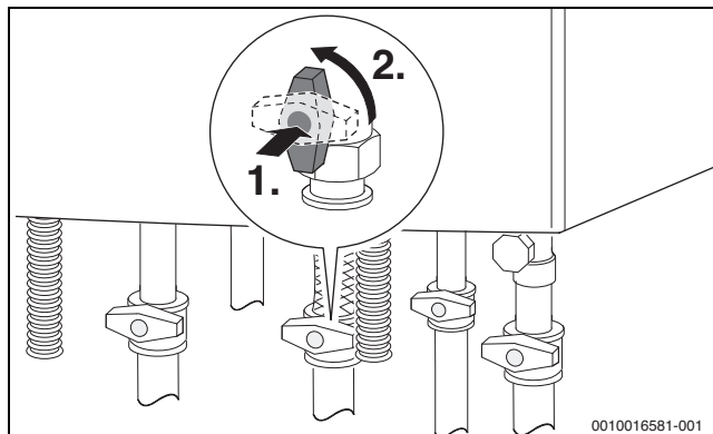
Мал. 5 Відкриття газового крана
